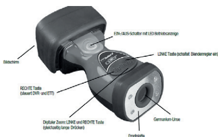
Wärmebildkamera
